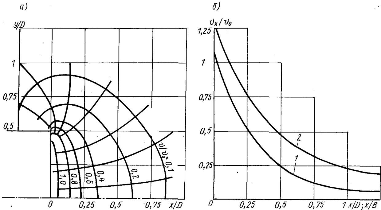
Рис. 8.1. Распределение скоростей в зоне действия всасывающих отверстий
