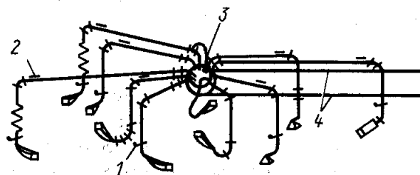
Рис. 9.3. Кустовая система с малогабаритным коллектором
