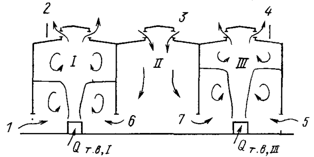
Рис. 5.5. Схема аэрации трехпролетного здания с тепловыделениями в крайних пролетах
