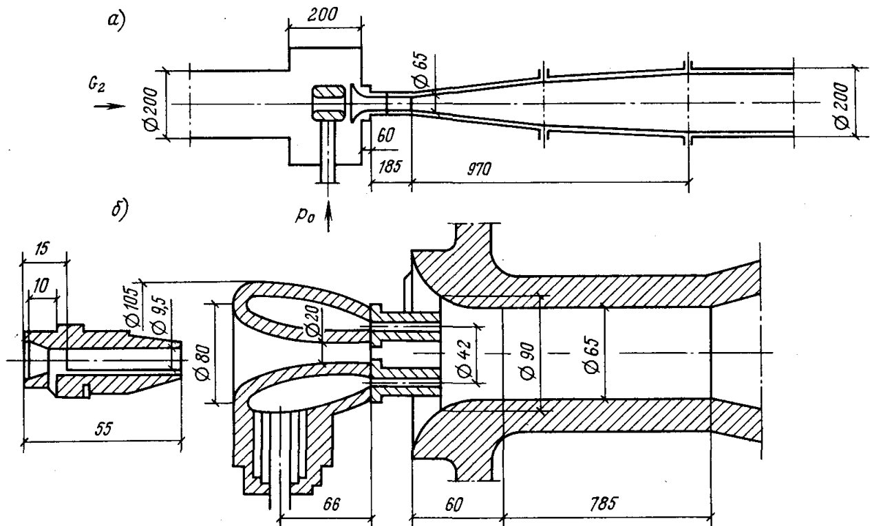
Рис. 10.9. Многоструйный эжектор
