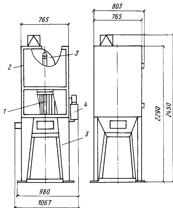
Рис. 4.17. Тканевый пылеуловитель АІ-БПШ
