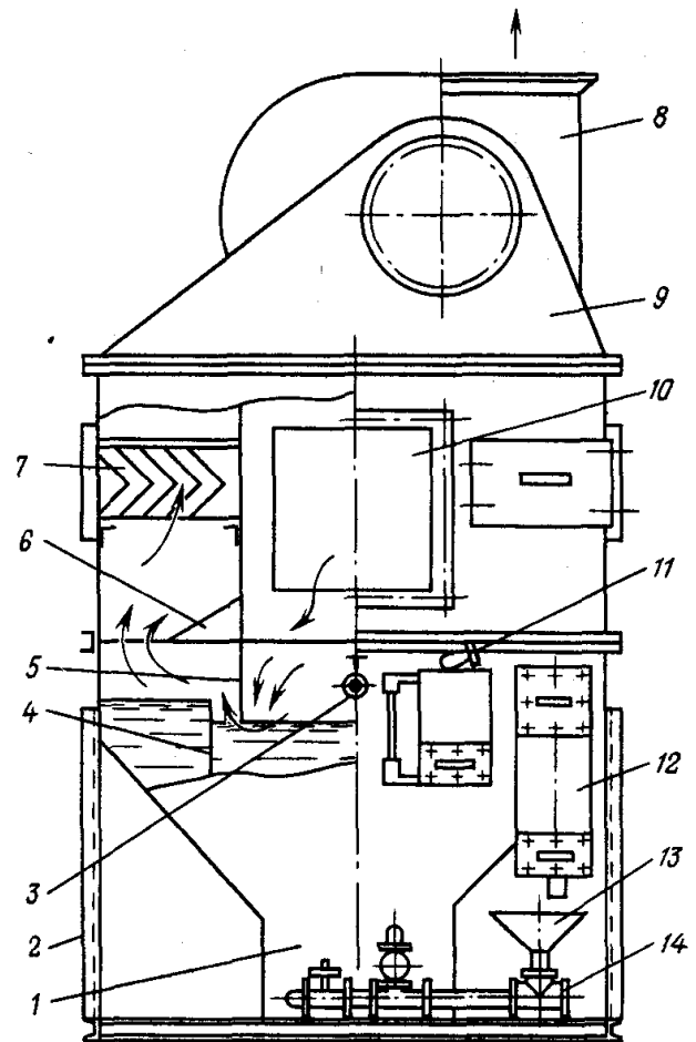
Рис. 4.13. Устройство пылеуловителя ПВМ
