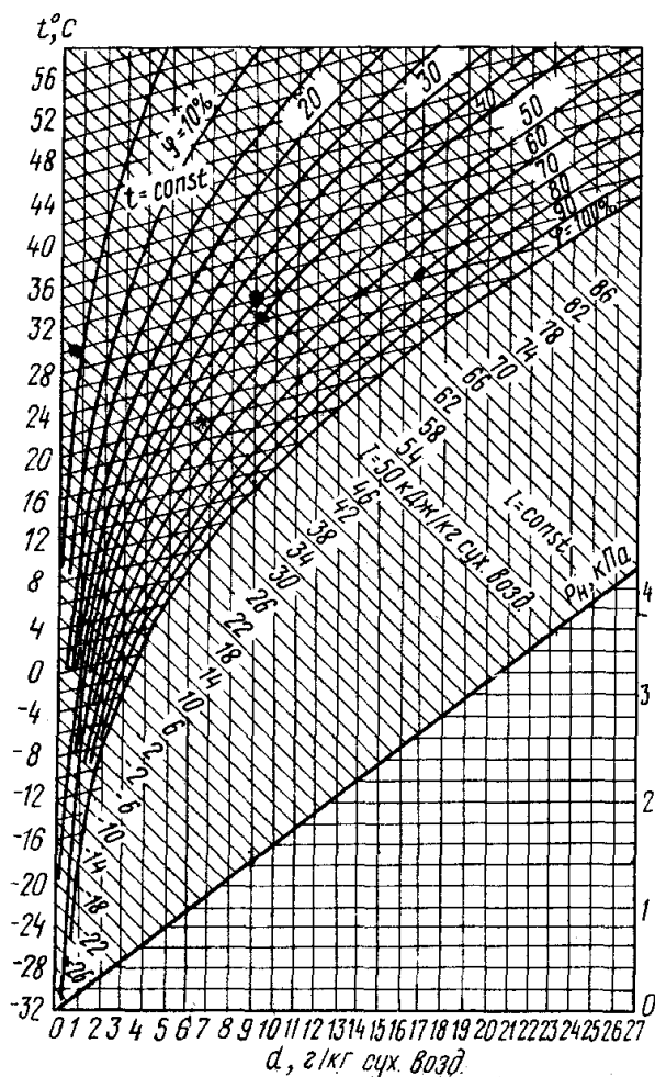
Рис. 1.1. I - d -диаграмма влажного воздуха
