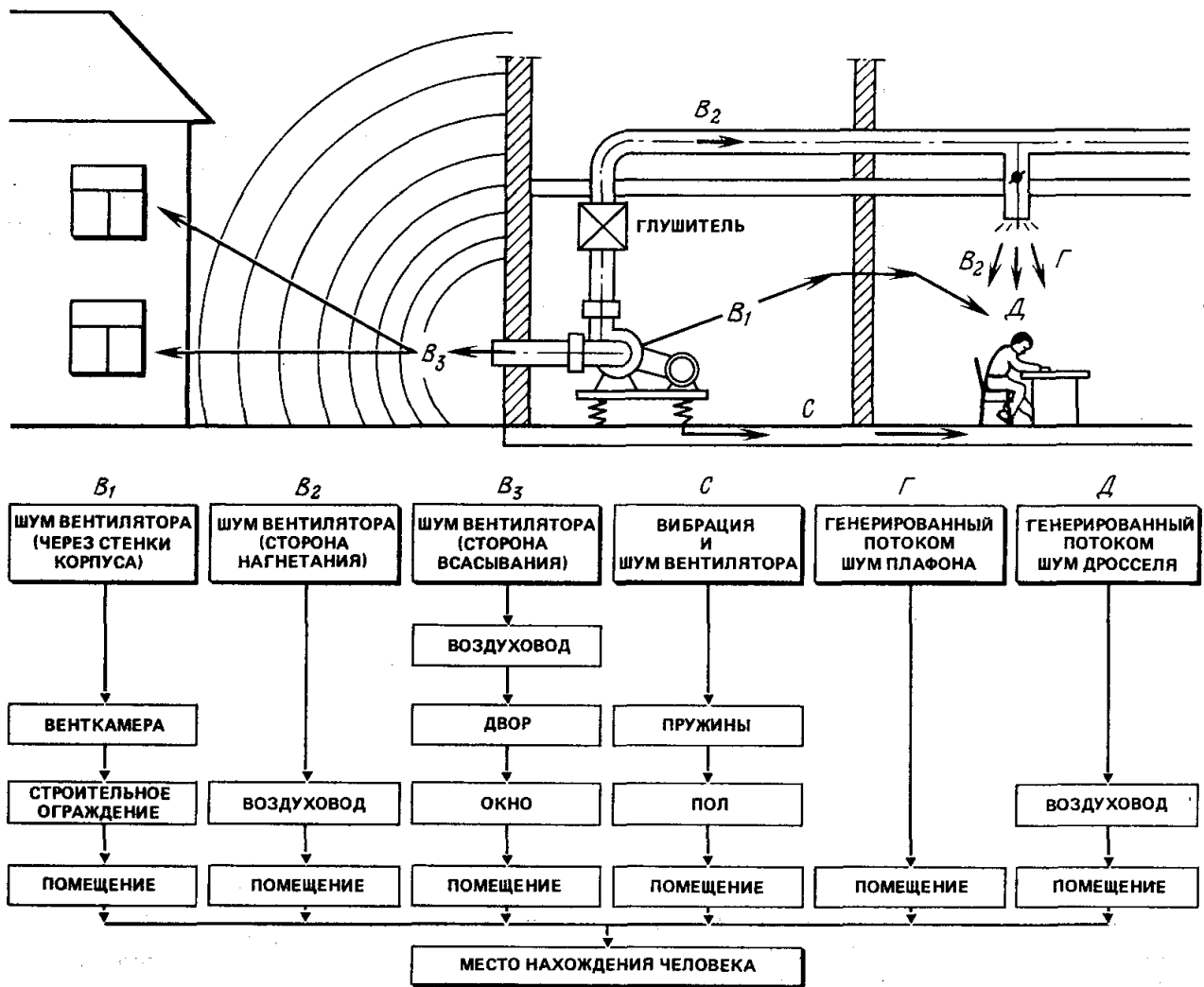
Рис. 12.1. Основные источники шума и пути распространения звука и вибрации
