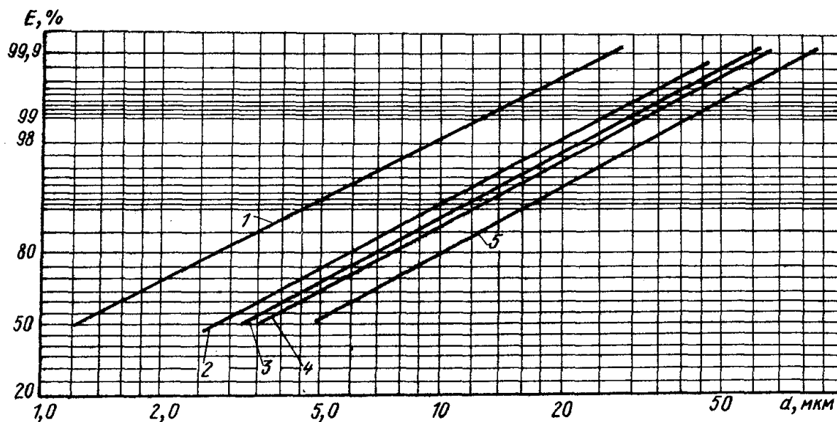
Рис. 4.10. Фракционная эффективность циклонов ВНИИОГАЗа
