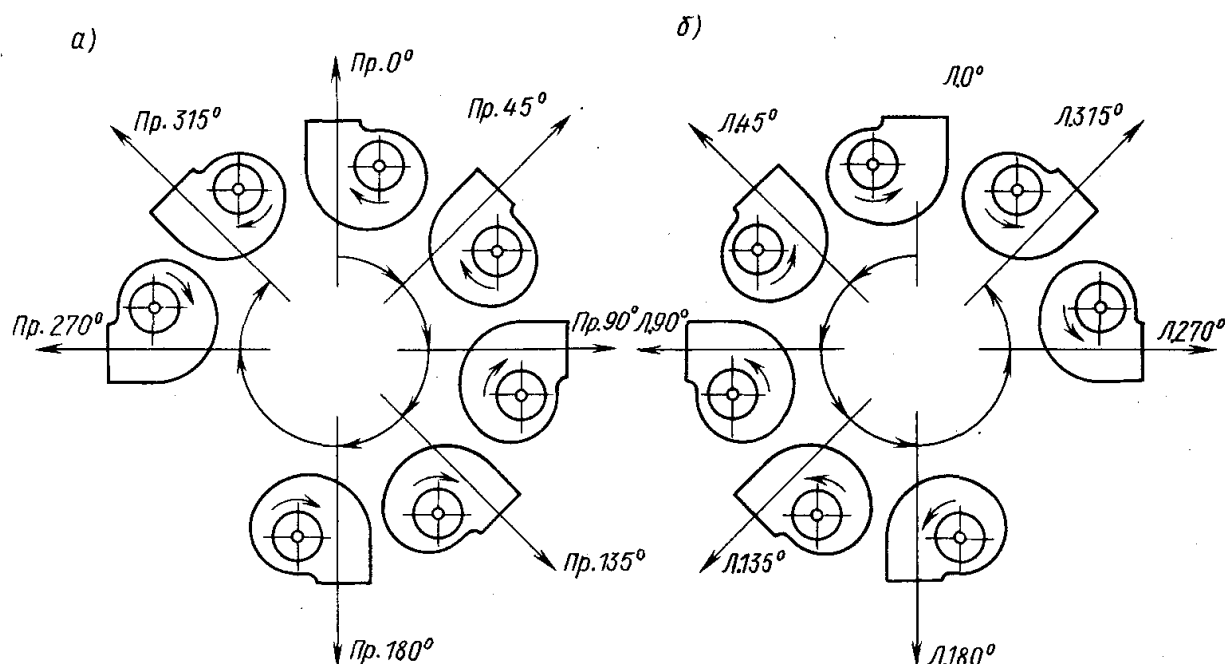
Рис. 11.6. Расположение корпусов радиальных вентиляторов правого (а) и левого (б) вращения
