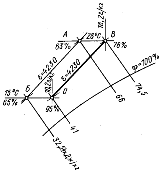
Рис. 14.10. К примеру 14.5
