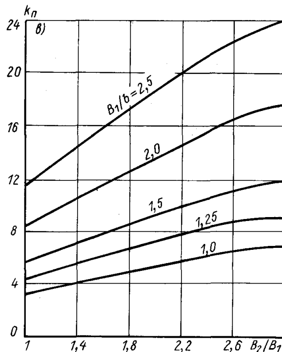
Рис. 8.11. Нижние отсосы
