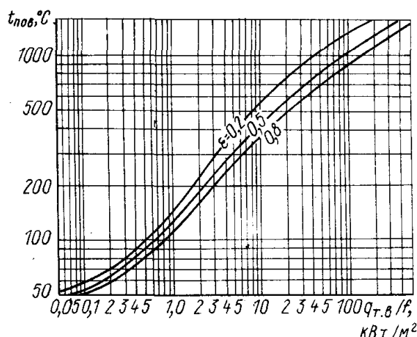
Рис. 5.9. Зависимость температуры поверхности источника тепловыделений от удельной теплонапряженности и степени черноты его поверхности ( f — площадь поверхности источника)
