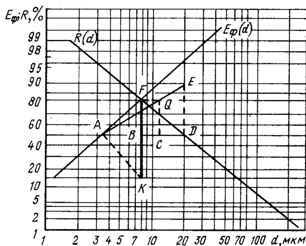
Рис. 4.12. К примеру расчета циклона ЦН-15 графоаналитическим методом
