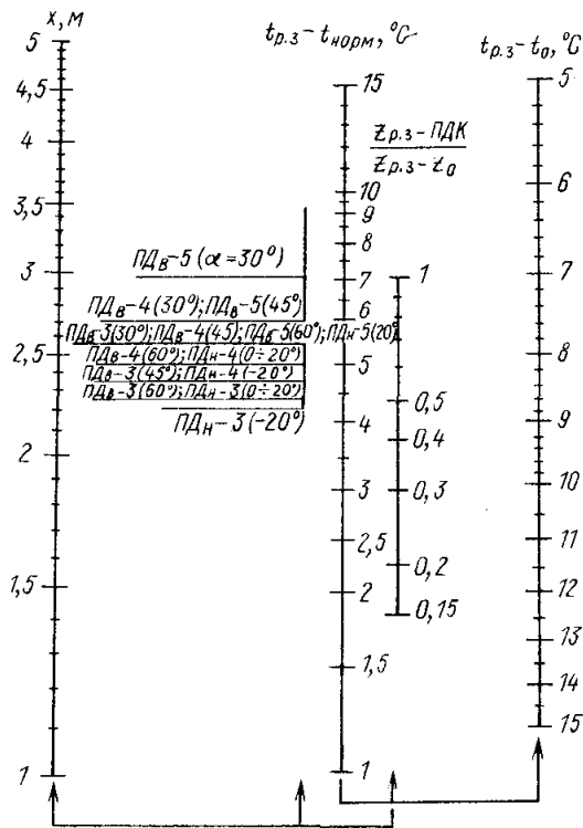
Рис. 6.13. Номограмма для определения типоразмера ПД
