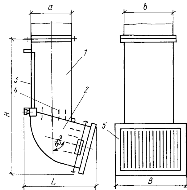
Рис. 6.5. Воздухораспределитель поворотный регулируемый типа ВП с присоединительным патрубком прямоугольного сечения – ВП1 и ВП2
