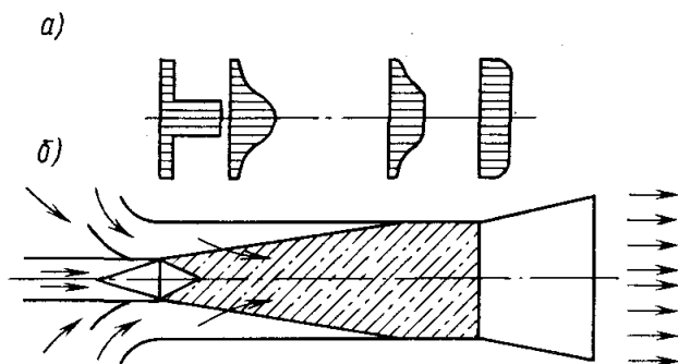
Рис. 10.1. Схема распределения скоростей воздуха по длине камеры смещения эжектора
