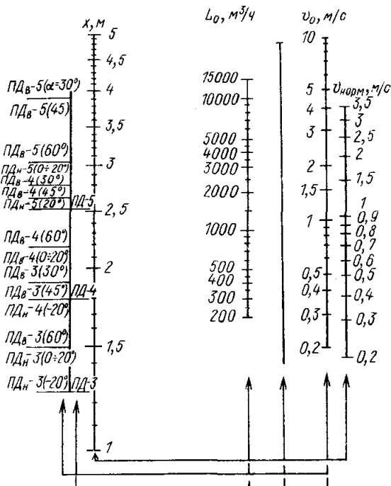
Рис. 6.14. Номограмма для определения расхода воздуха на ПД
