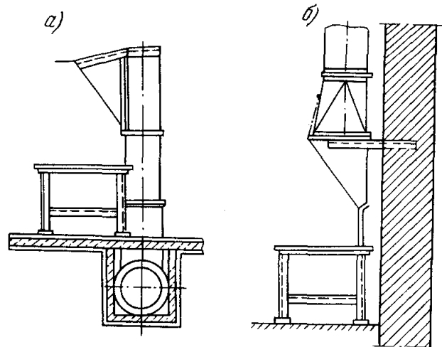
Рис. 8.7. Панели равномерного всасывания у стационарных постов сварки
