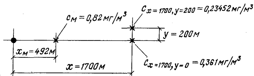
Рис. 13.5. К примеру 13.2
