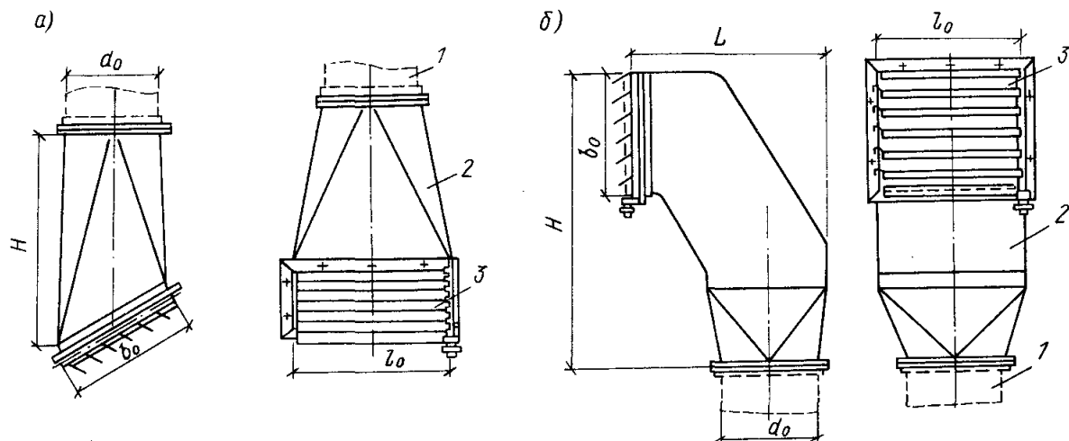
Рис. 6.4. Душирующие патрубки типа ПД
