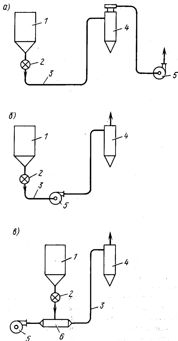
Рис. 9.3. Кустовая система с малогабаритным коллектором
