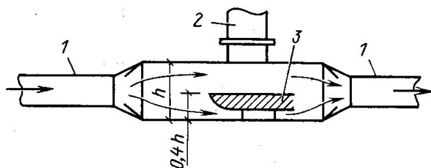
Рис. 9.2. Приемная коробка
