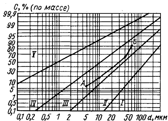
Рис. 4.2. Классификационная номограмма пылей I–V–зоны классификационных групп пылей по их дисперсности
