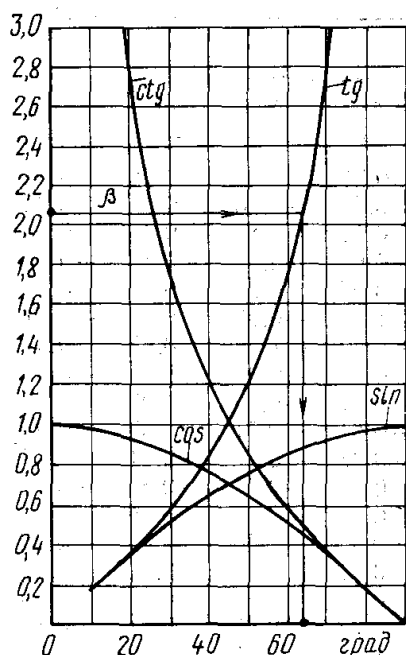
Рис. 2.4. К определению значений тригонометрических функций и угла \beta = \arctg(\operatorname{ctg} L \cdot \cos A_{c.o.})
