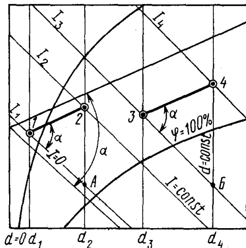
Рис. 1.4. Построение процесса на I - d -диаграмме для случая 3
