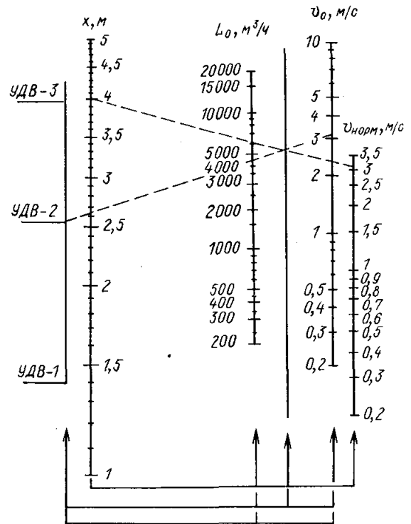
Рис. 6.10. Номограмма для определения расхода воздуха на УДВ
