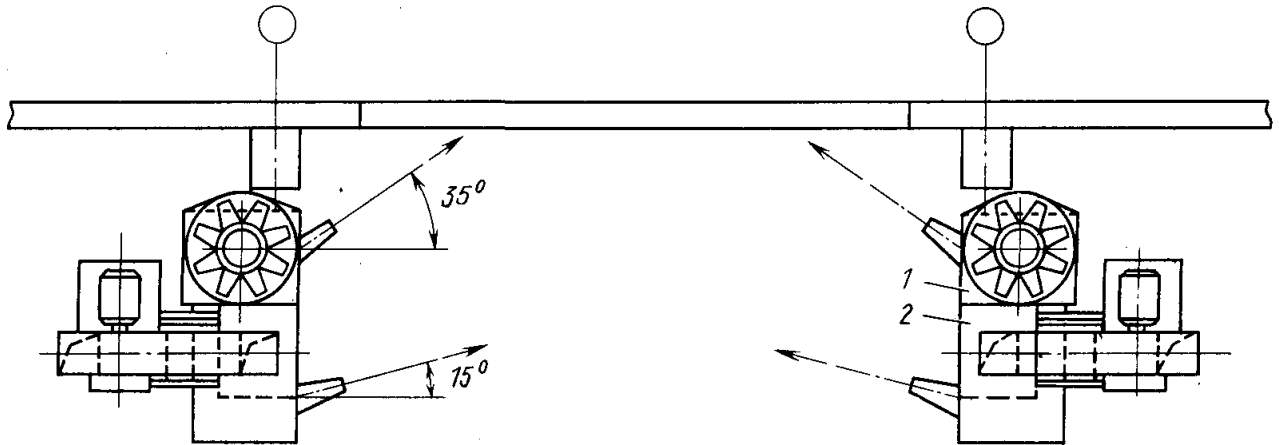
Рис. 7.5. Комбинированная воздушно-тепловая завеса
