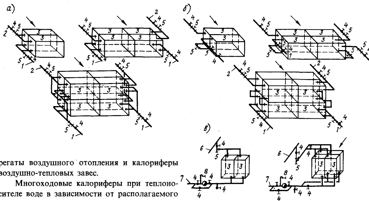
Рис. 11.5. Схемы подвода теплоносителя к калориферам
