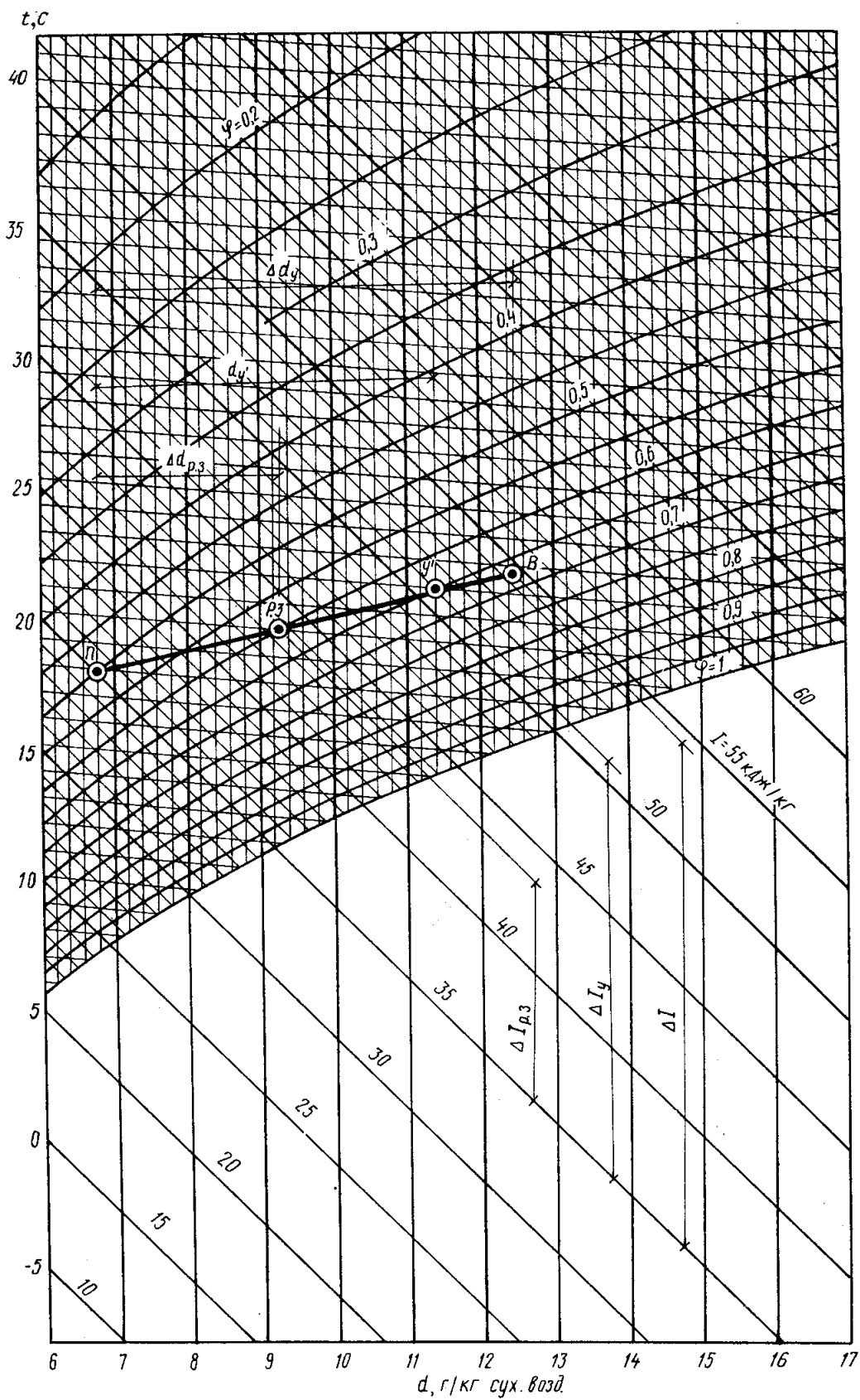
Рис. 2.11. Графический расчет вентиляции с использованием I-d -диаграммы
