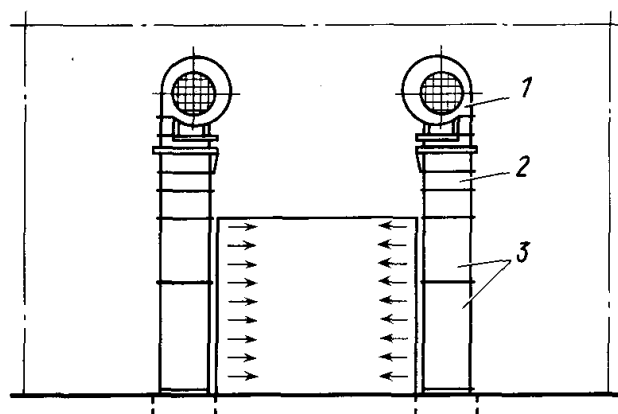
Рис. 7.1. Двусторонняя воздушно-тепловая завеса шибберного типа
