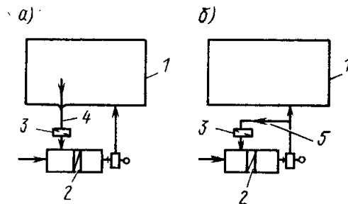
Рис. 11.4. Схемы приточной установки или кондиционера, работающих с частичной рециркуляцией воздуха (а) либо только на наружном воздухе (б)
