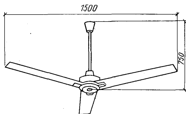
Рис. 6.8. Вентилятор потолочный типа ВПК-15 «Союз»
