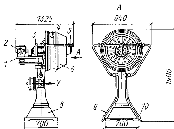
Рис. 6.7. Поворотный аэратор ПАМ-24
