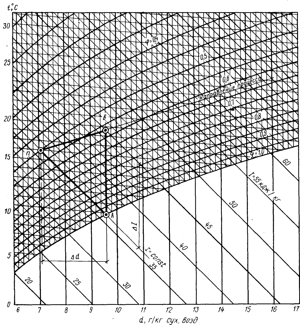
Рис. 2.10. Построение процесса совместного выделения влаги и теплоты на I-d -диаграмме
