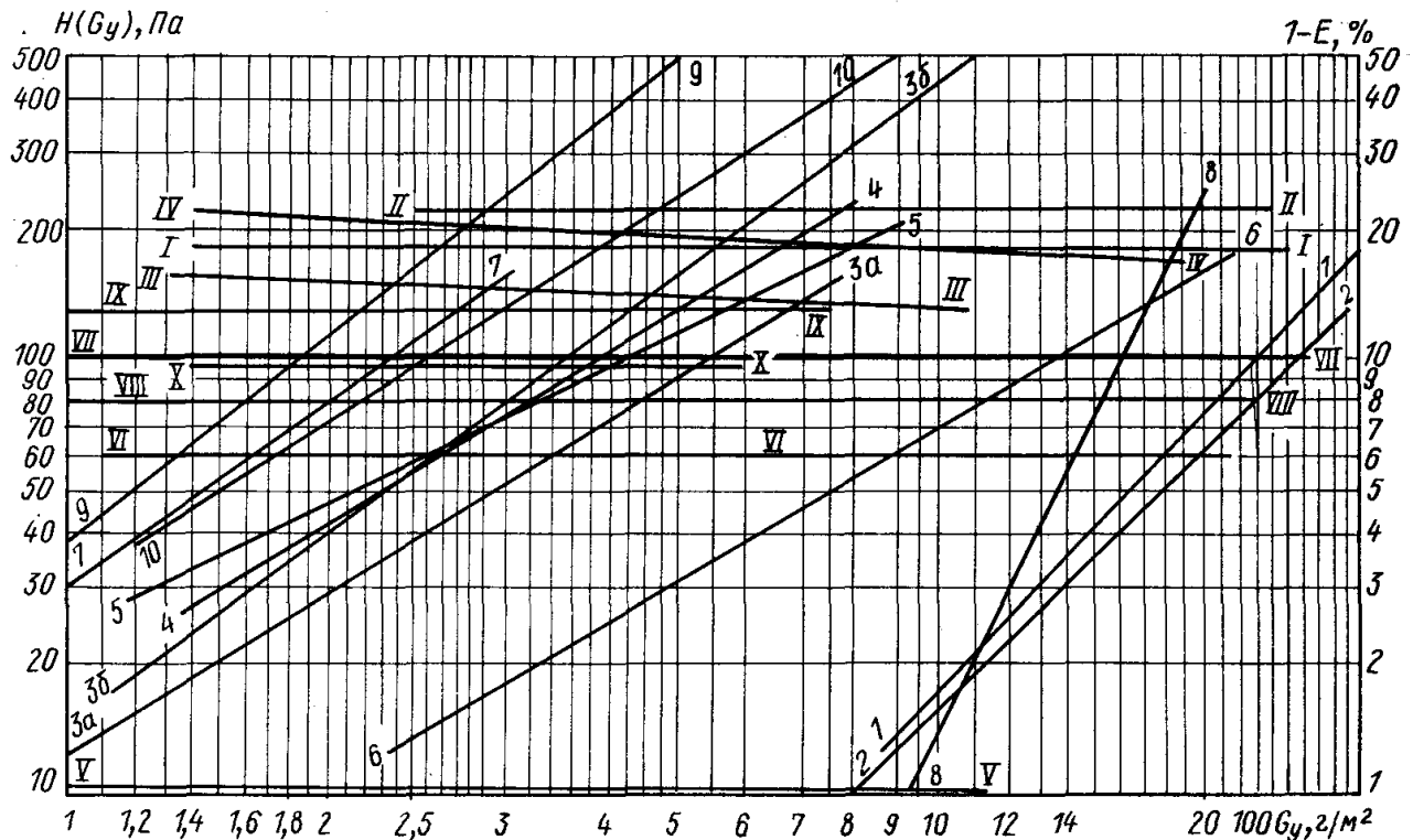
Рис. 4.4. Пылевая характеристика фильтра и фильтрующих материалов
