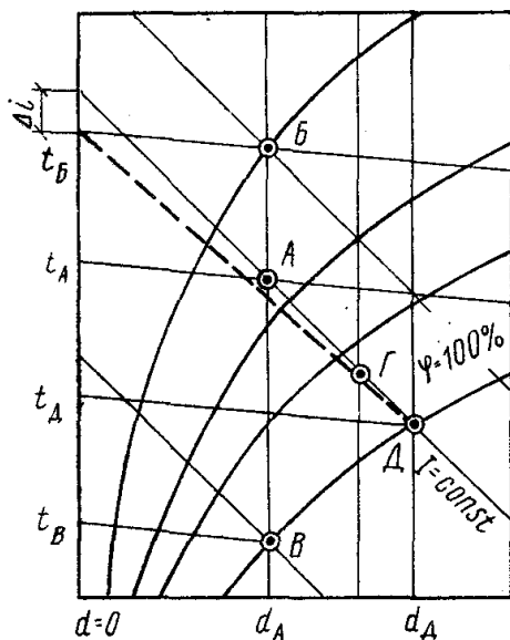
Рис. 1.2. Построение процесса на I - d -диаграмме для случая 1
