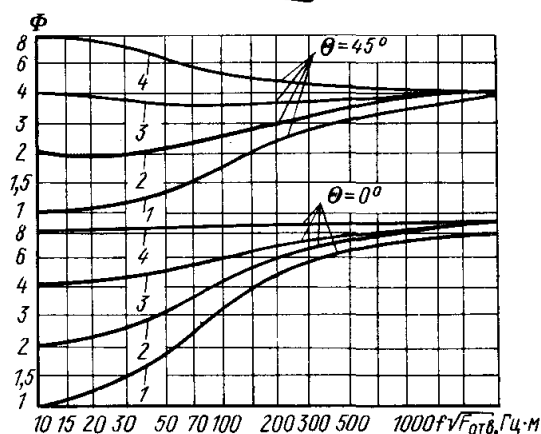
Рис. 12.4. Схема возможного размещения вентиляционных отверстий (решеток) (а) и кривые коэффициента направленности излучения \Phi источника шума (б)
