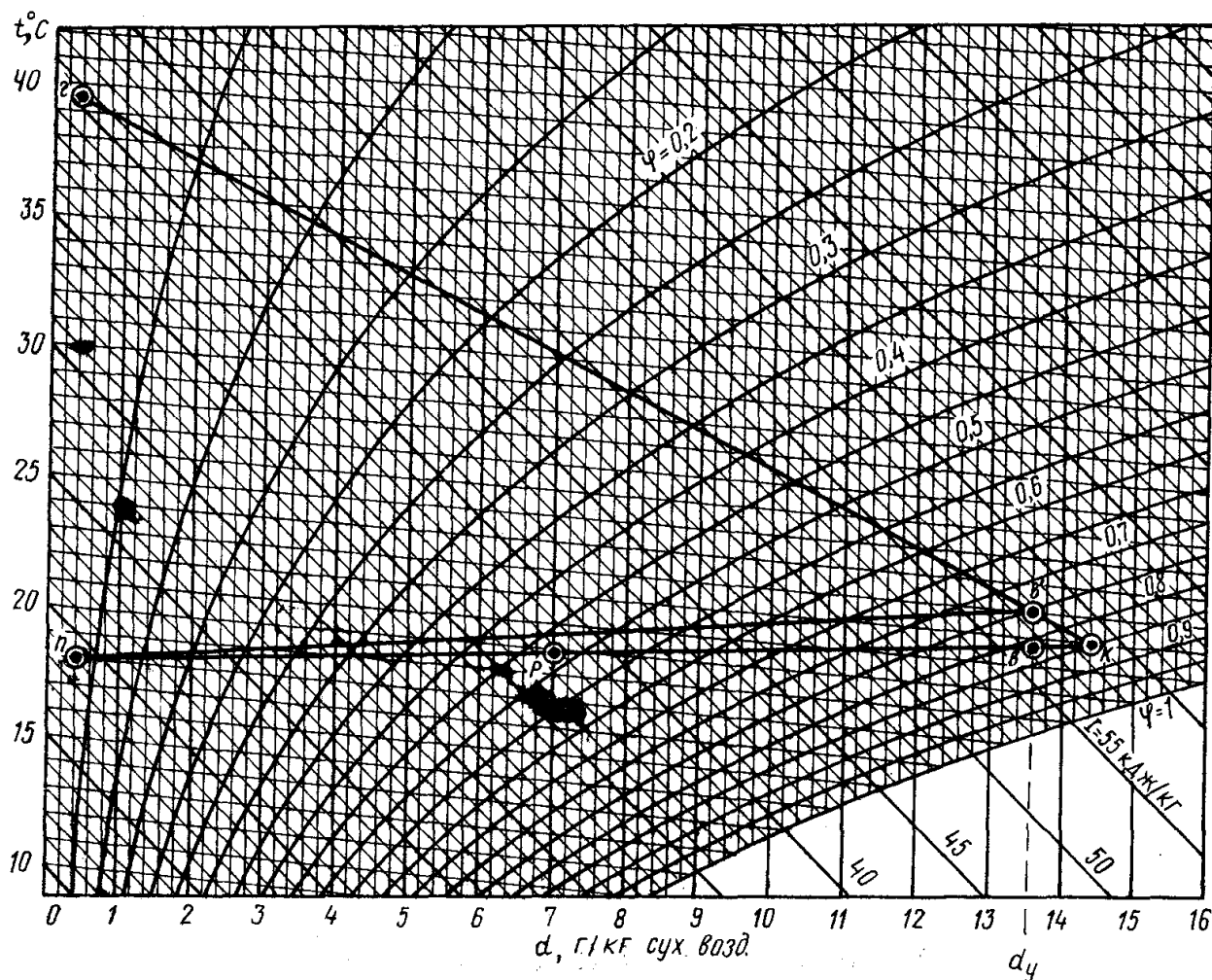
Рис. 2.13. Ход расчета продувки верхней зоны помещения на I-d -диаграмме
