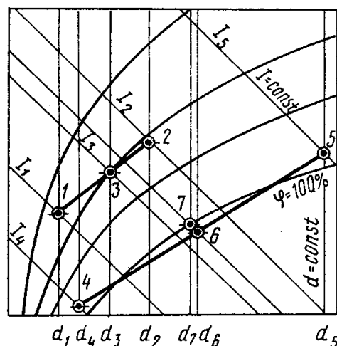
Рис. 1.3. Построение процесса на I - d -диаграмме для случая 2
