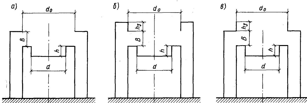
Рис. 8.9. Кольцевые бортовые отсосы а - обычный; б - заглубленный; в - с экраном
