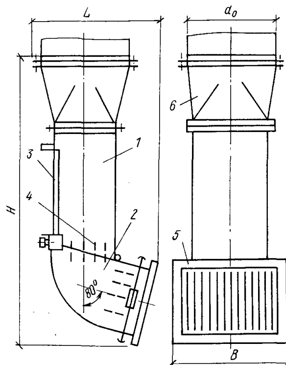
Рис. 6.6. Воздухораспределитель поворотный регулируемый типа ВП с присоединительным патрубком круглого сечения – ВП3 и ВП4
