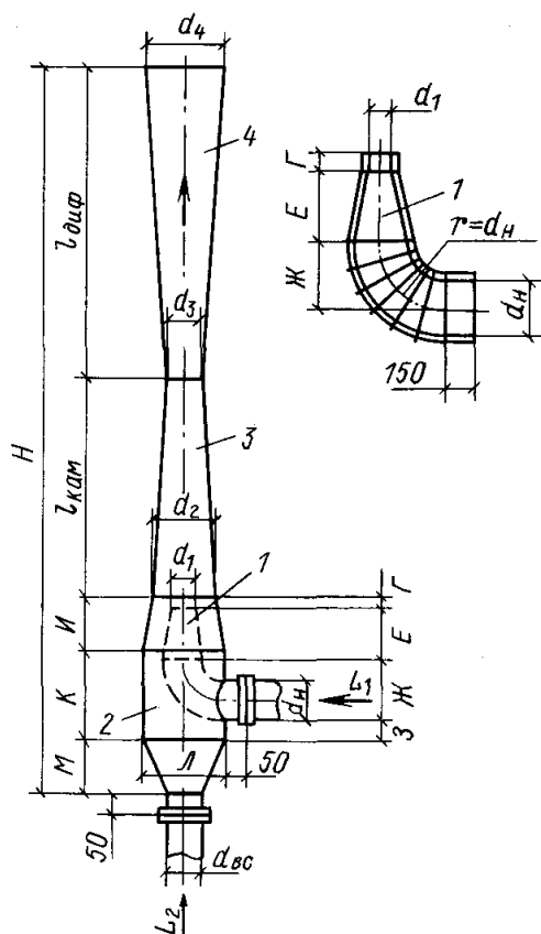
Рис. 10.2. Эжектор низкого давления
