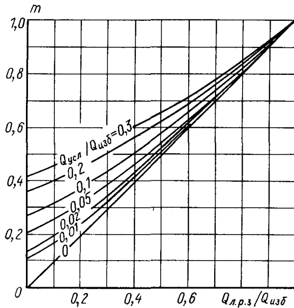
Рис. 5.3. Номограмма для определения высоты расположения температурного перекрытия Z (при c_p = 1 кДж/(кг·°C); T_{p.з} = 298 К; \rho_{p.з} = 1,18 кг/м³). Ключ: G = 100 кг/с; Q_k = 1000 кВт; n = 10 ; Z + Z_n = 7,6 м
