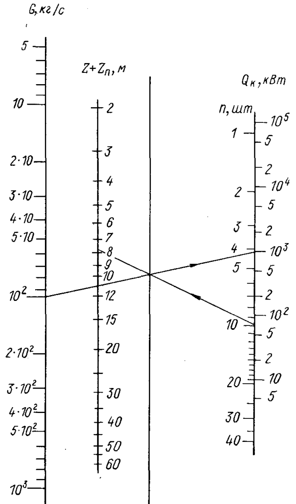
Рис. 5.3. Номограмма для определения высоты расположения температурного перекрытия Z (при c_p = 1 кДж/(кг·°C); T_{p.з} = 298 К; \rho_{p.з} = 1,18 кг/м³). Ключ: G = 100 кг/с; Q_k = 1000 кВт; n = 10 ; Z + Z_n = 7,6 м
