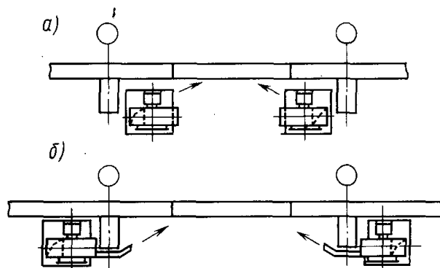
Рис. 7.2. Размещение завес
