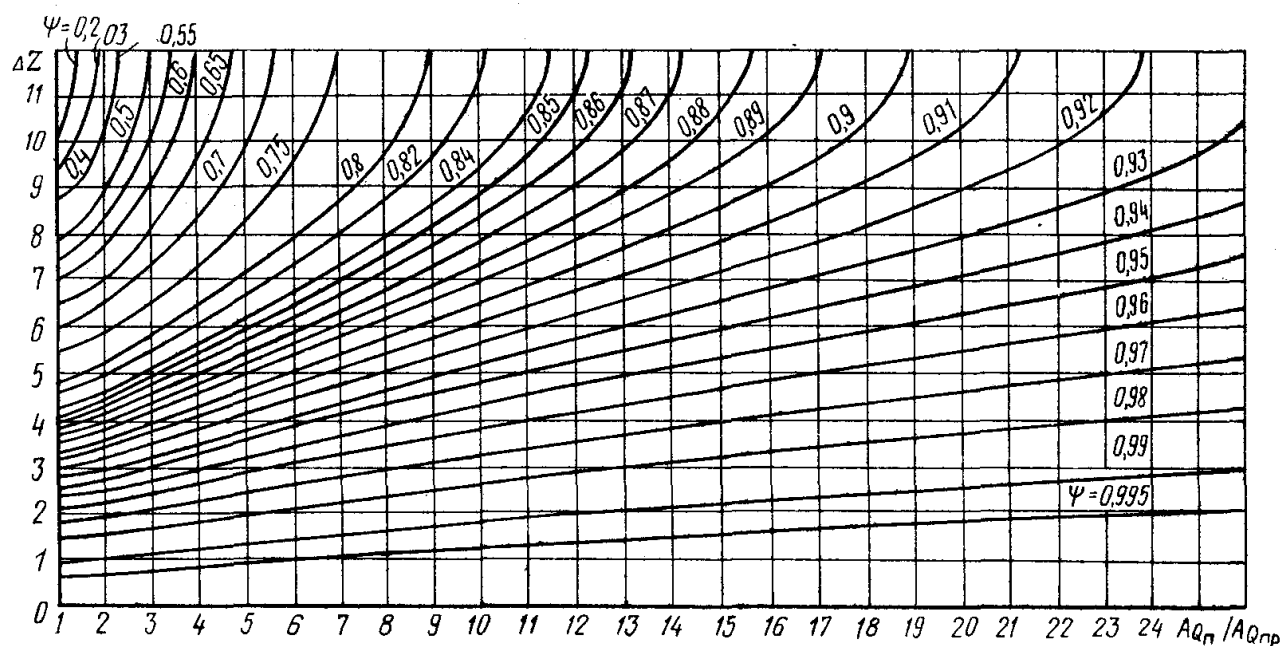
Рис. 2.7. Коэффициент \psi
