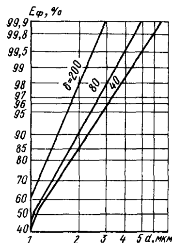
Рис. 4.15. Зависимость фракционной эффективности E_\phi пылеуловителей ПВМ от уровня воды (см. рис. 4.13).
