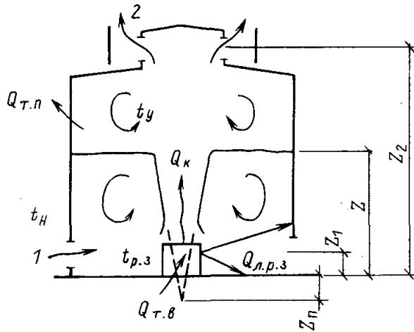
Рис. 5.1. Схема аэрации однопролетного здания 1 и 2 — номера проемов
