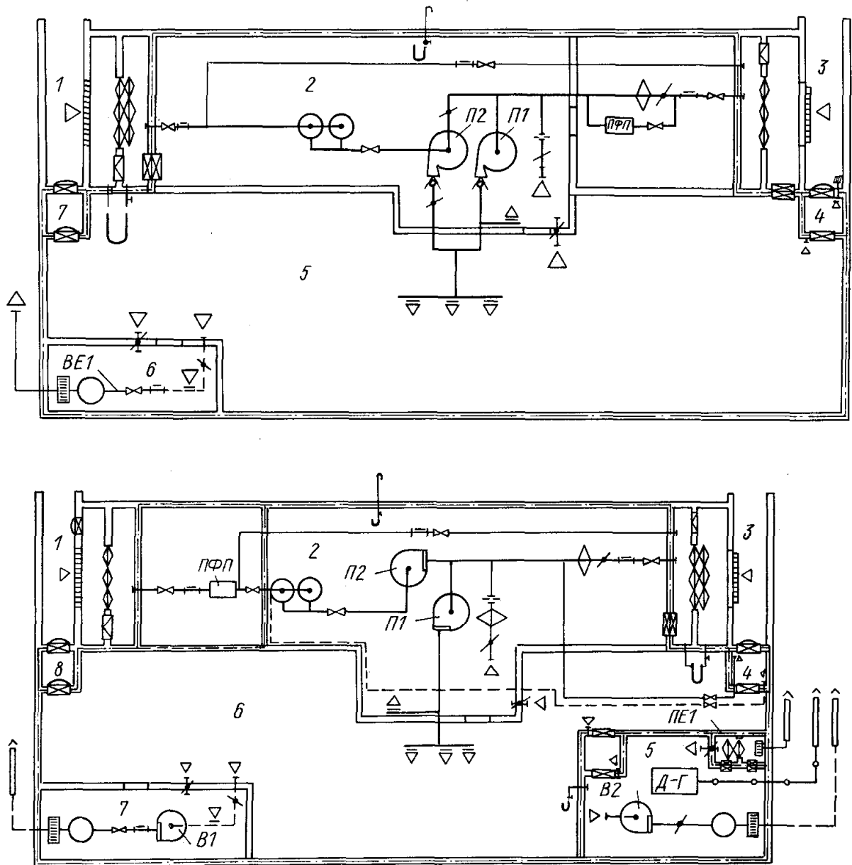
Рис. 14.1. Принципиальная схема вентиляции убежища, оборудованного электроручными вентиляторами для режимов вентиляции I и II
