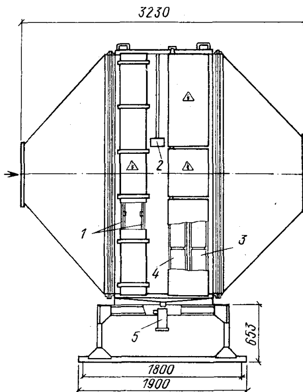
Рис. 4.16. Двухкаскадный электрический уловитель масляных аэрозолей ЭФУ202
