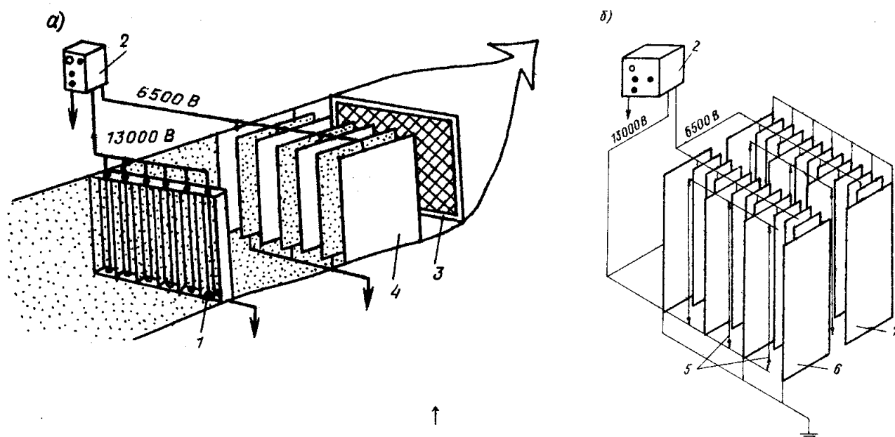
Рис. 4.6. Принципиальная схема двухзонного электрофилтра
