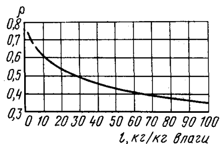
Рис. 2.9. Зависимость коэффициента прорыва тепла и влаги \beta от удельного расхода воздуха l , удаляемого из-под зонта или завесы
