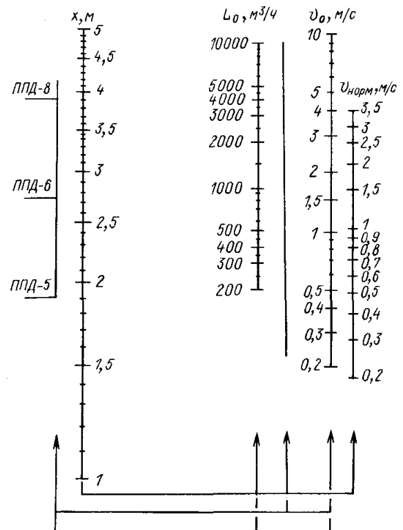
Рис. 6.12. Номограмма для определения расхода воздуха на ППД
