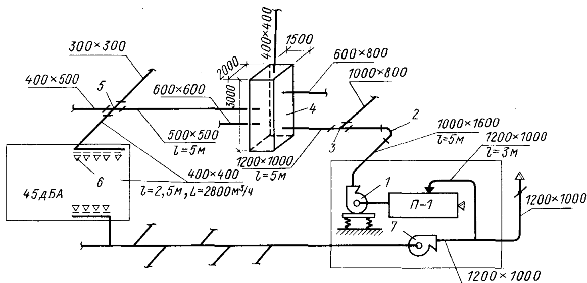
Рис. 12.6. Схема расчетной ветви воздуховодов 1 - приточный вентилятор; 2 - плавный поворот; 3 - тройник; 4 - камера статического давления; 5 - крестовина; 6 - жалюзий- ные решетки; 7 - рециркуляционный вентилятор
