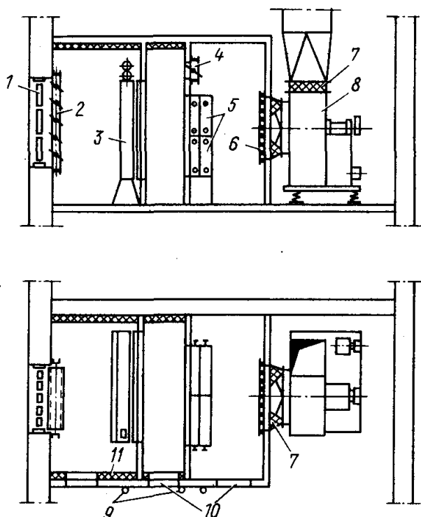
Рис. 11.3. Компоновка приточной камеры
