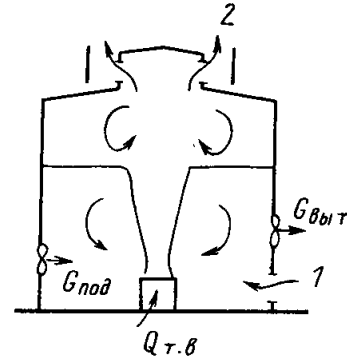
Рис. 5.8. Схема аэрации здания, оборудованного местной механической вентиляцией
