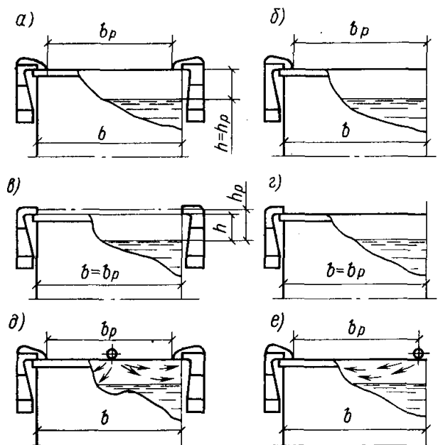
Рис. 8.8. Бортовые отсосы от ванн
