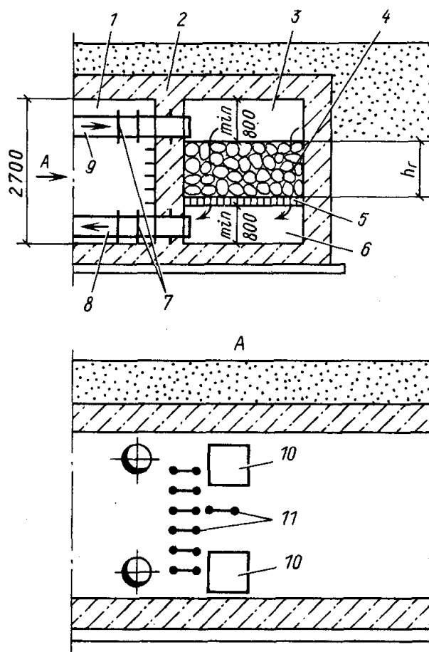
Рис. 14.5. Гравийный охладитель
