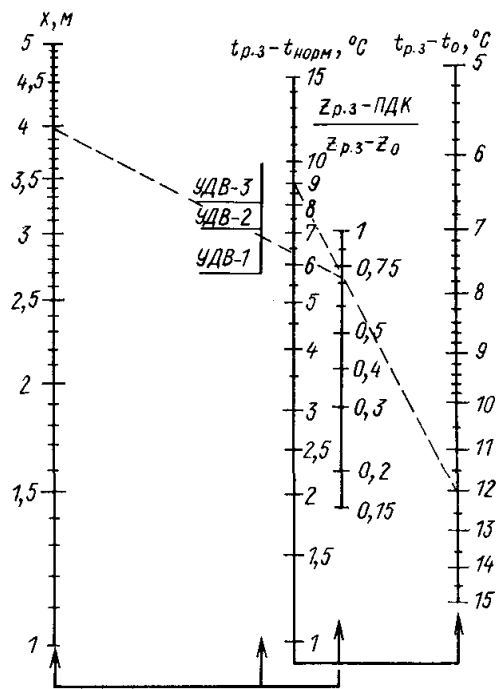
Рис. 6.9. Номограмма для определения типоразмера УДВ
