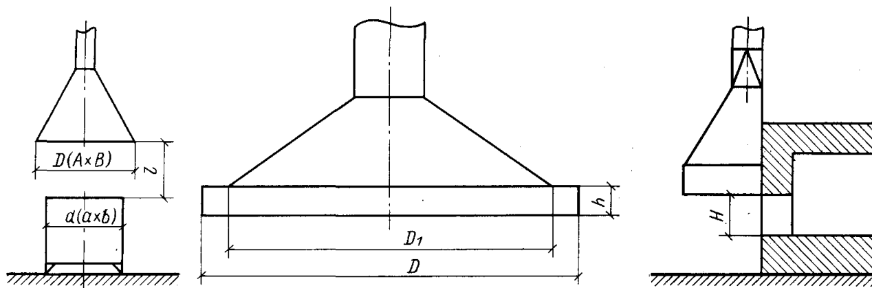
Рис. 8.3. Вытяжной зонт над теплоисточником
