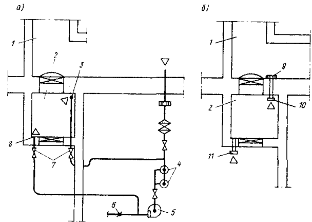
Рис. 14.6. Продувка тамбура входа
