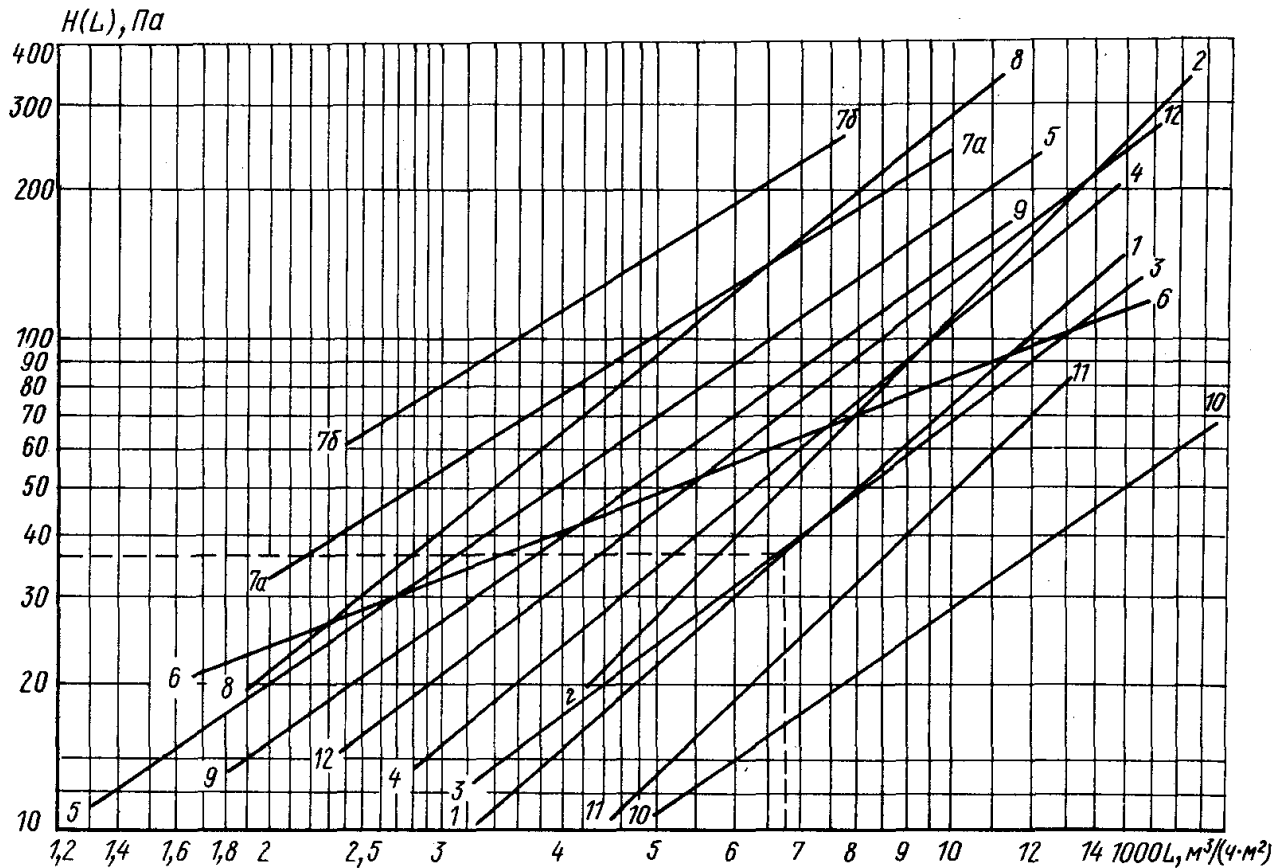
Рис. 4.3. Аэродинамические характеристики фильтров и фильтрующих материалов
