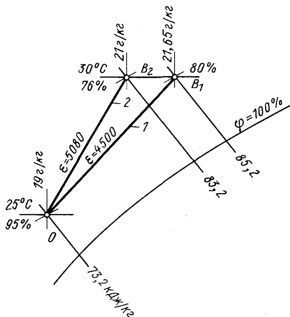
Рис. 14.8. I - d -диаграмма 1-к примеру 14.2; 2-к примеру 14.3
