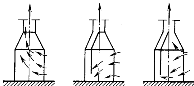
Рис. 8.17. Укрытия шкафного типа
