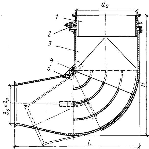
Рис. 6.3. Поворотный душирующий патрубок типа ППД
