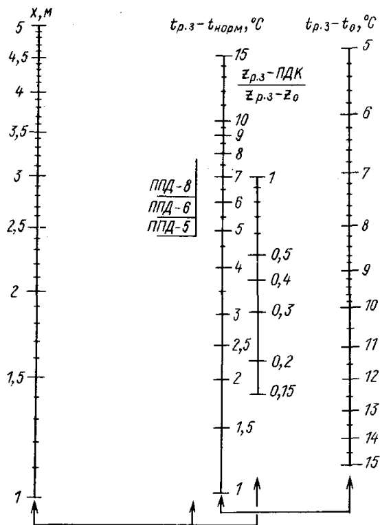
Рис. 6.11. Номограмма для определения типоразмера ППД
