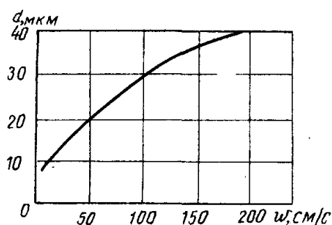
Рис. 4.8. Зависимость граничного размера оседающих частиц от средней скорости турбулентного потока в пылеосадочной камере
