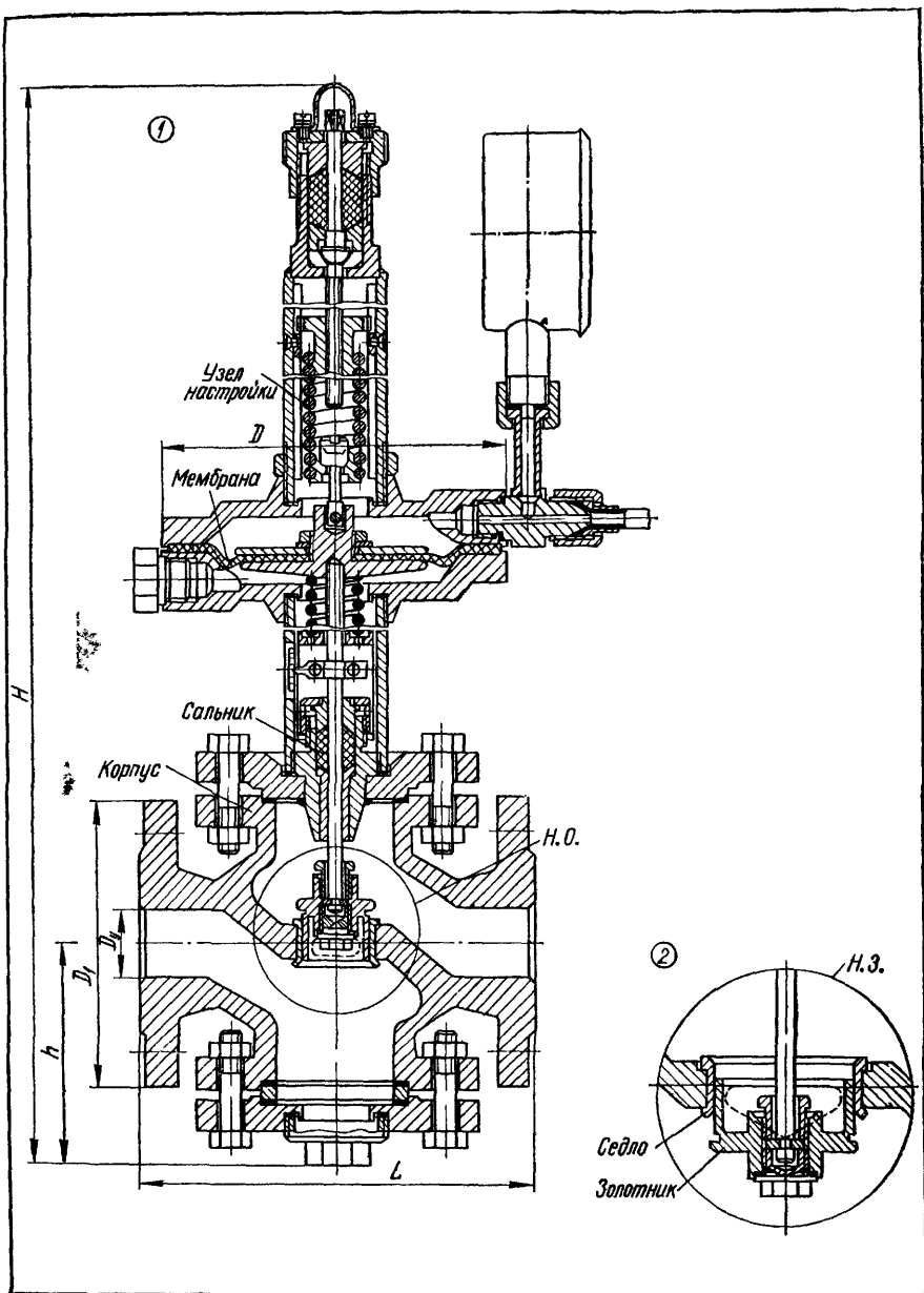
Лист IX.1. Клапан типа ПК-1:
