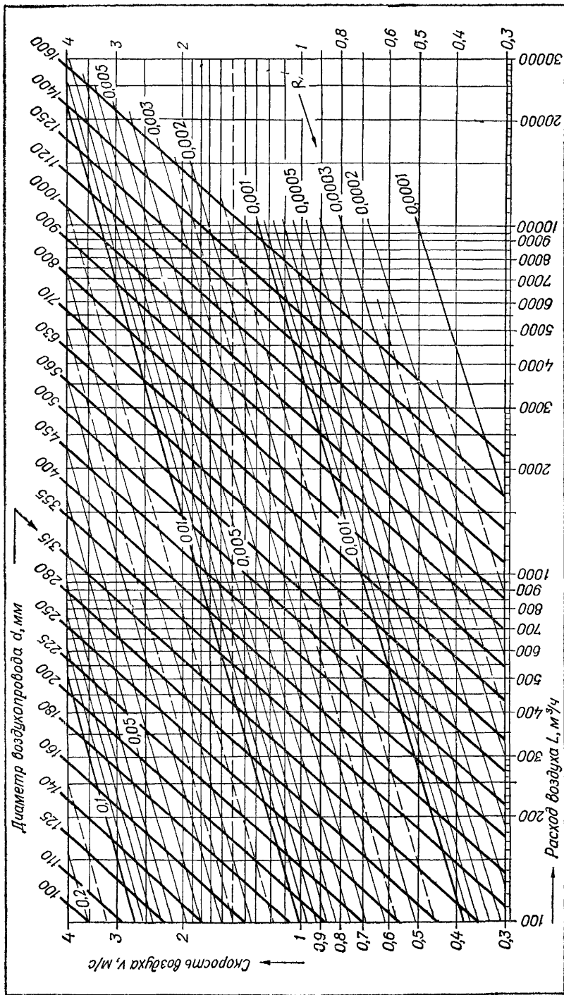
Лист VII.8. Номограмма для расчета круглых стальных воздухопроводов при расходах воздуха от 100 до 10 000 м 3 /ч и скорости воздуха от 0,3 до 4 м/с (при K = 0,1 , \gamma = 1,2 кг/м 3 ).
