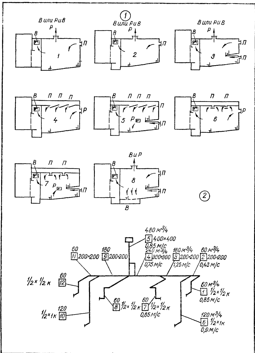
Лист VII.1. Схема вентиляции зрительных залов (рис. 1) и расчетная схема к примеру VII.2 (рис. 2):
