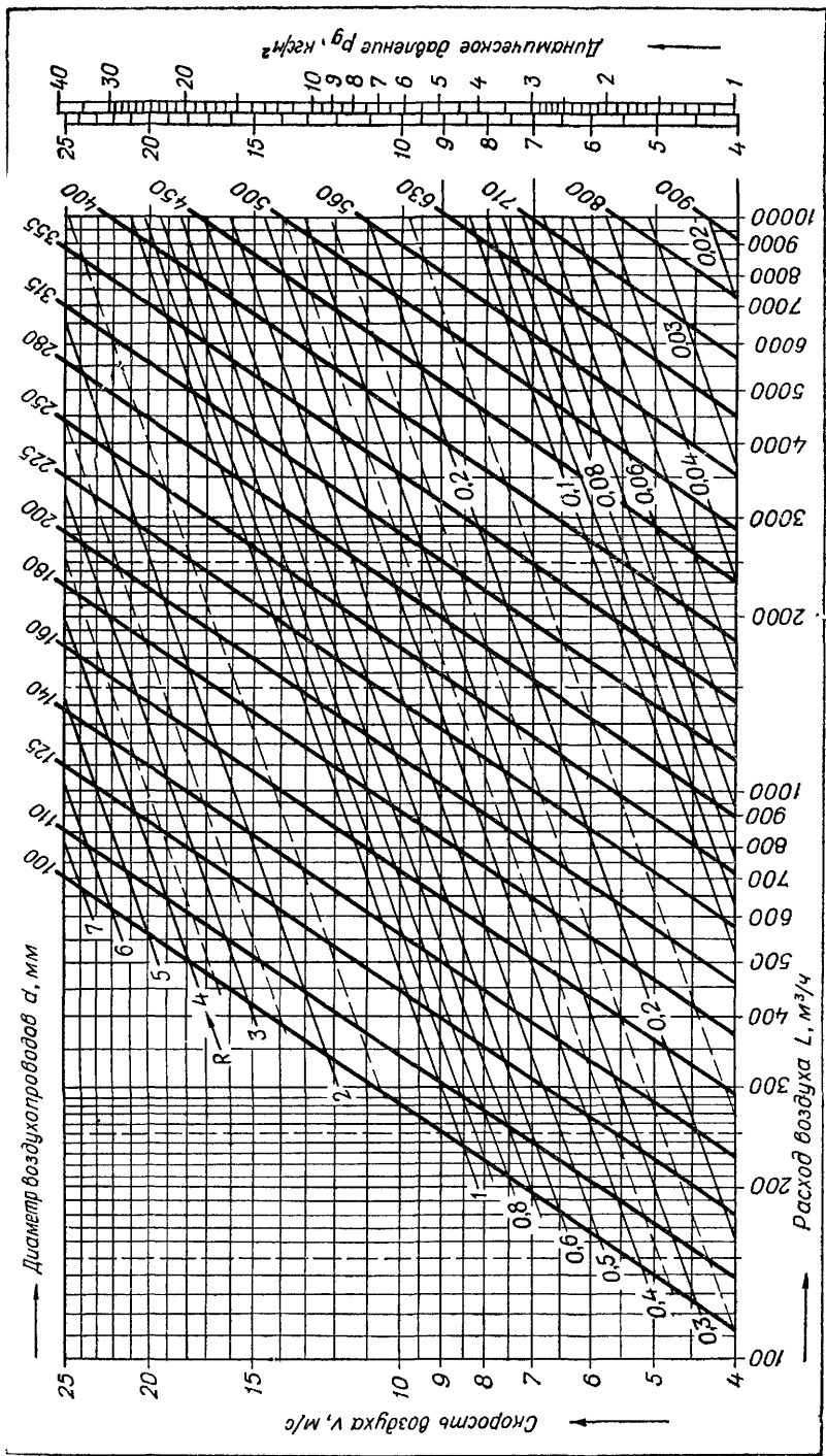
Лист VII.9. Номограмма для расчета круглых стальных воздухопроводов при расходах воздуха от 100 до 10 000 м 3 /с и скорости воздуха от 4 до 25 м/с (при K = 0,1 ; \gamma = 1,2 кг/м 3 ).
